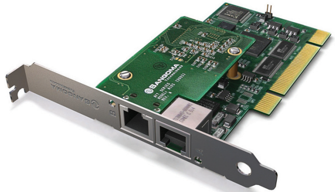
La tarjeta A102 T1/E1/J1 de 2 puertos con interfaz PCI disponible.
